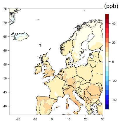
(d) G5NR-Chem
