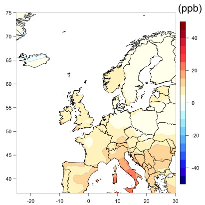
(b) GEOSCCM
