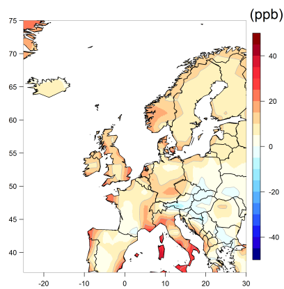
(e) MOCAGE
